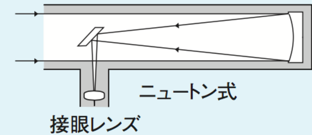
反射式望遠鏡
