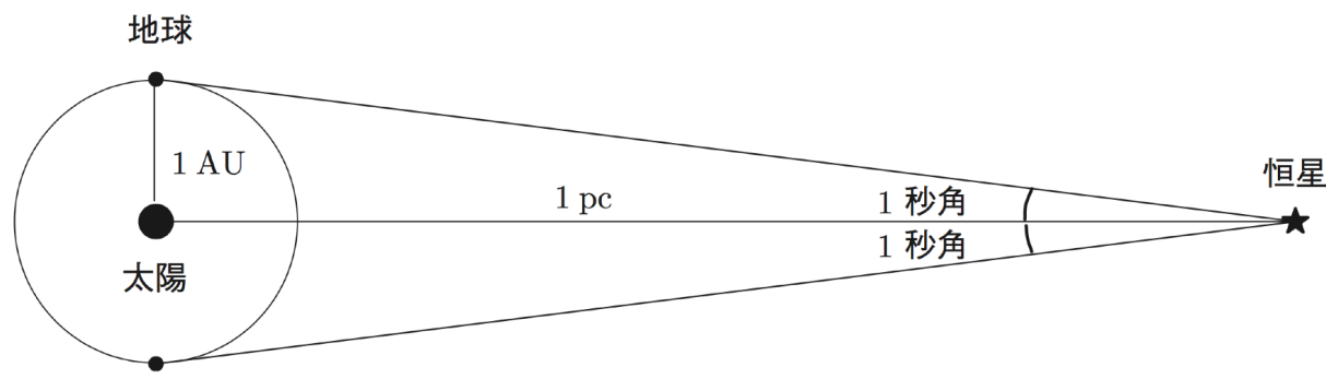
図 A.2 距離パーセク (pc) の定義. 地球から見る星の位置が半年で 2 秒角ずれる場所までの距離を 1 pc とする.
