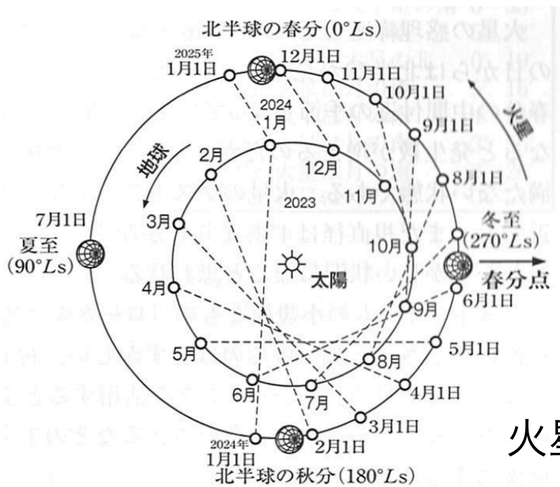
図1 2024年 地球と火星の位置
