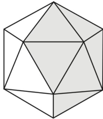
正 20 面体
