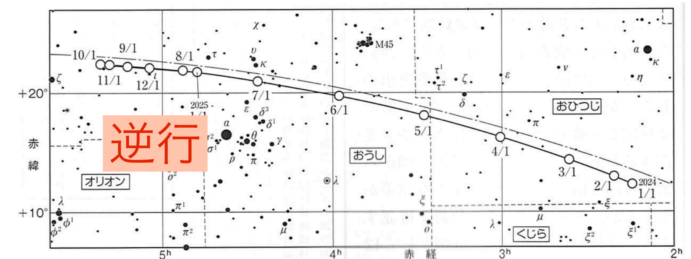
図2 2024年 星座間の木星の動き（毎月1日の位置）
