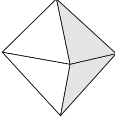
正 8 面体
