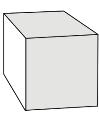
立方体
