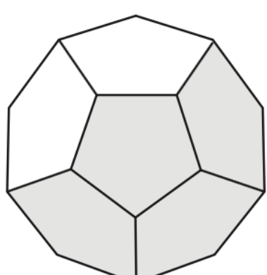
正 12 面体
