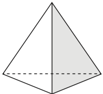
正 4 面体
