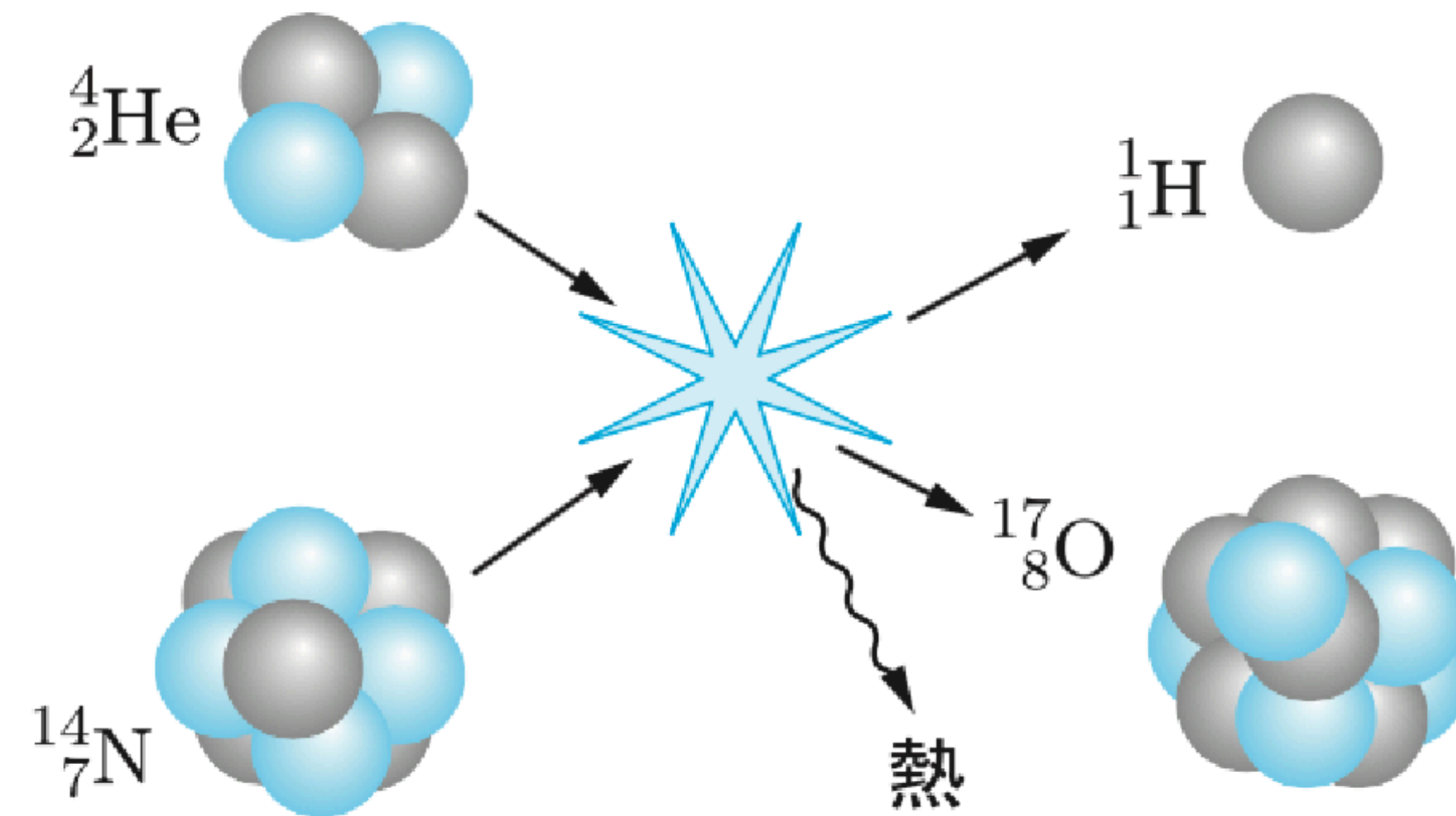
(b) 核反応
