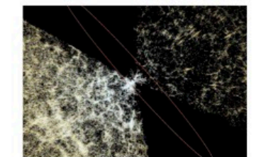
宇宙の大規模構造：銀河の集団である銀河団がつかって、泡状の構造を形成します。ひとつの泡のサイズは3億光年。宇宙で一番大きな構造です。
